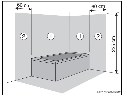
Fig. 6 Áreas de protección
