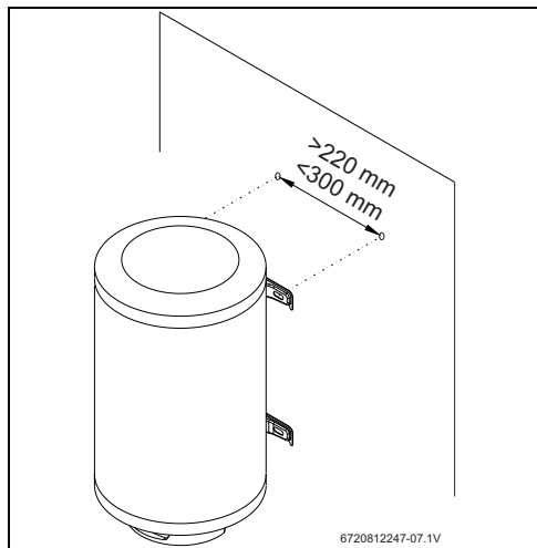
Fig. 7 Instalación en posición vertical
