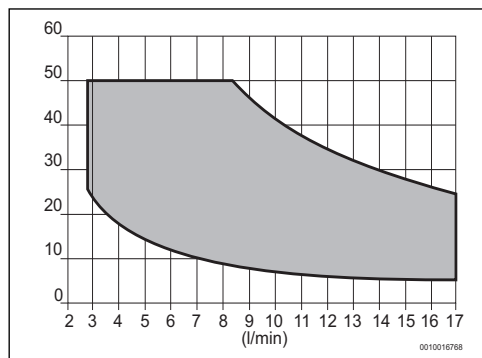
Fig. 29 Modelo 17 litros
