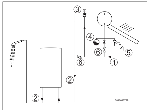
Fig. 18 Sistema solar
