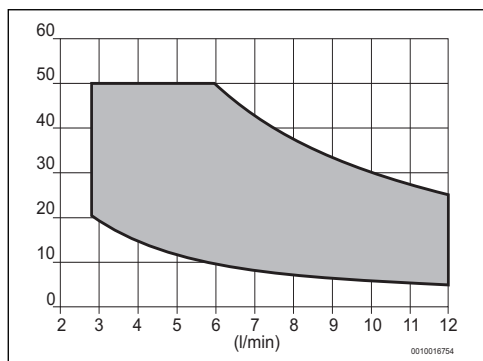
Fig. 27 Modelo 12 litros
