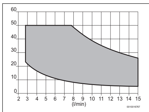
Fig. 28 Modelo 15 litros
