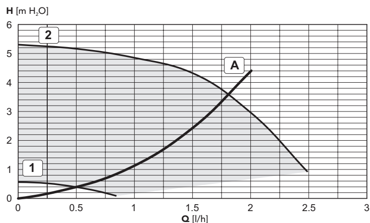
fig. 29 - Pérdida de carga/altura manométrica bomba BLUEHELIX TECH 18/25 A
