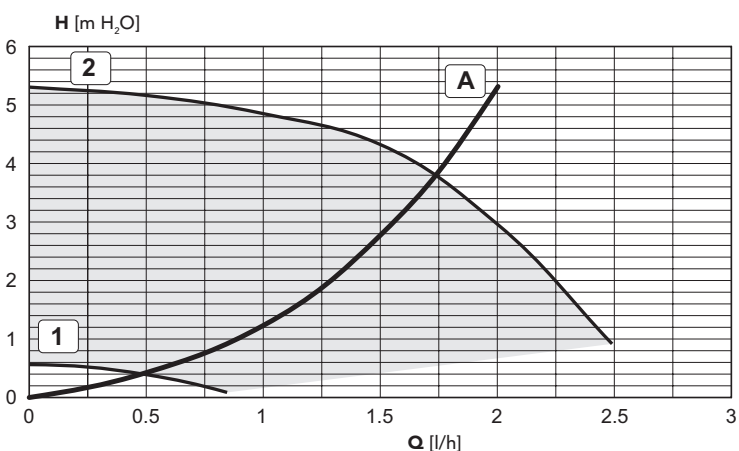
fig. 30 - Pérdida de carga/altura manométrica bomba BLUEHELIX TECH 35 A
