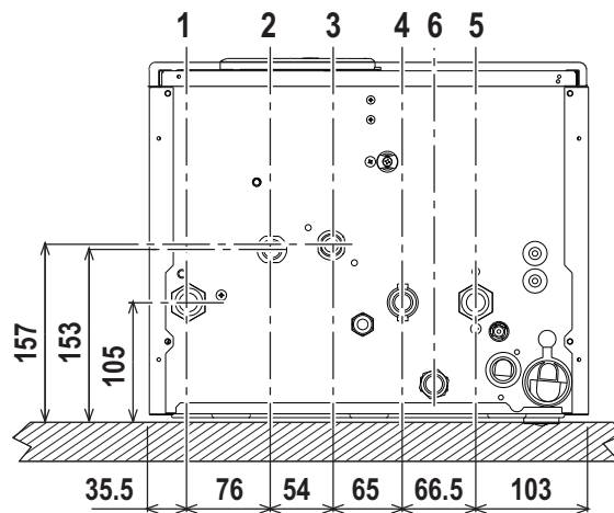
fig. 13 - Conexiones hidráulicas
