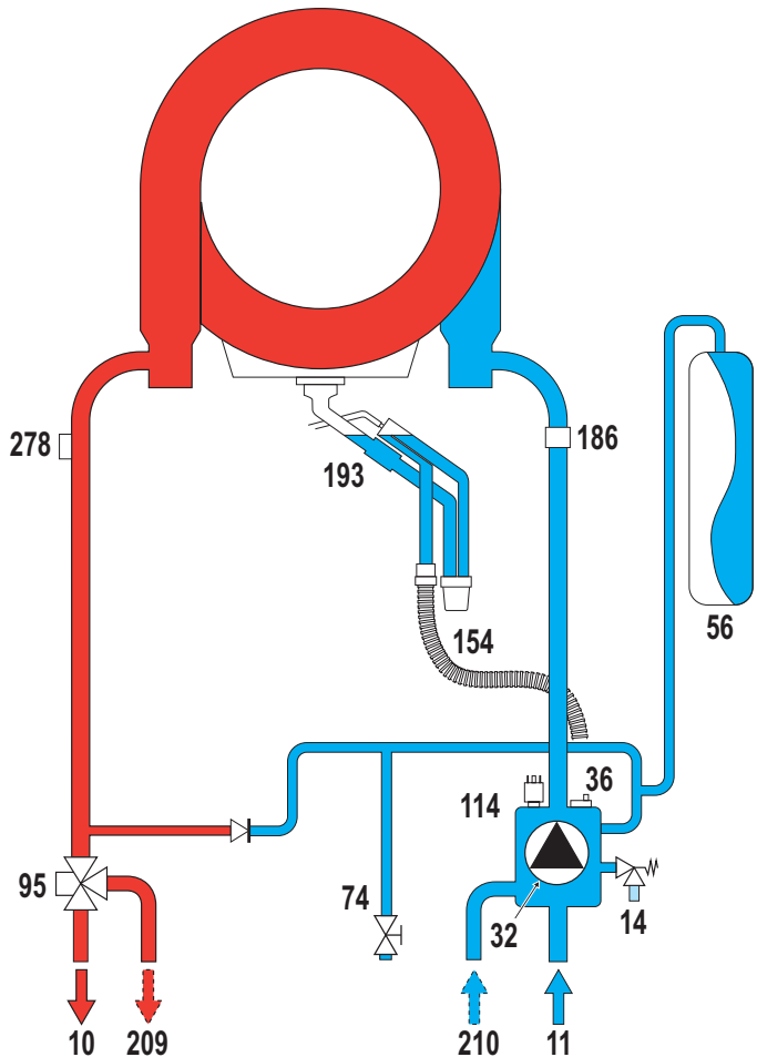
fig. 28 - Circuito hidráulico
