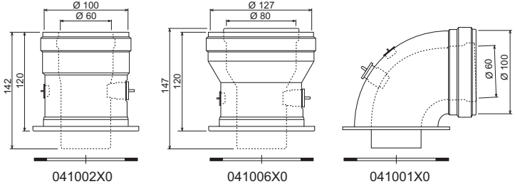
fig. 17 - Accesorios iniciales para conductos coaxiales
